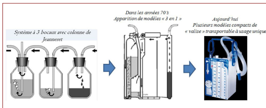
Figure 2. « Valise » transportable à usage unique, qui applique dans un même dispositif le principe des 3 boccas.
